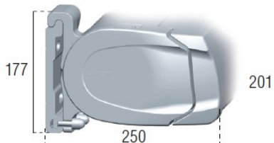
Instalación frontal | Wall mounting
