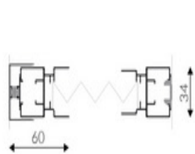
SECCCIÓN HORIZONTAL 1 HOJA
