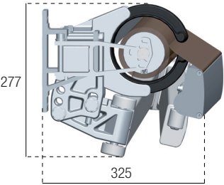
Instalación frontal | Wall mounting
