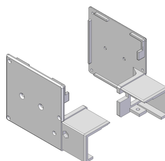
Soportes polea y tapas guía
