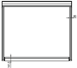
Vista dall'alto Top view
