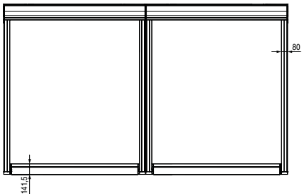
Vista dall'alto (3 profili guida) Top view (3 guide profiles)
