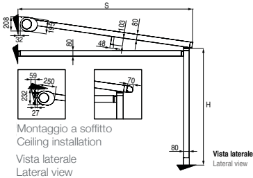
MODULO DOPPIO DOUBLE MODULE
